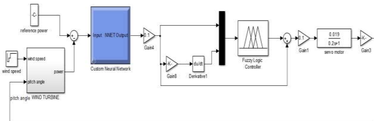
الشكل (5) نموذج آلية التحكم بزواوية انحراف شفرات العنفة الريحية
