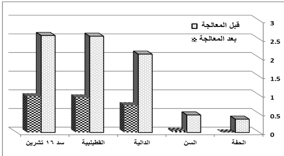
الشكل (9): قيم تراكيز الحموض الدبالية (HA) المقاسة في عينات مياه خام وعينات بعد خلطها مع الفحم الفعال.
