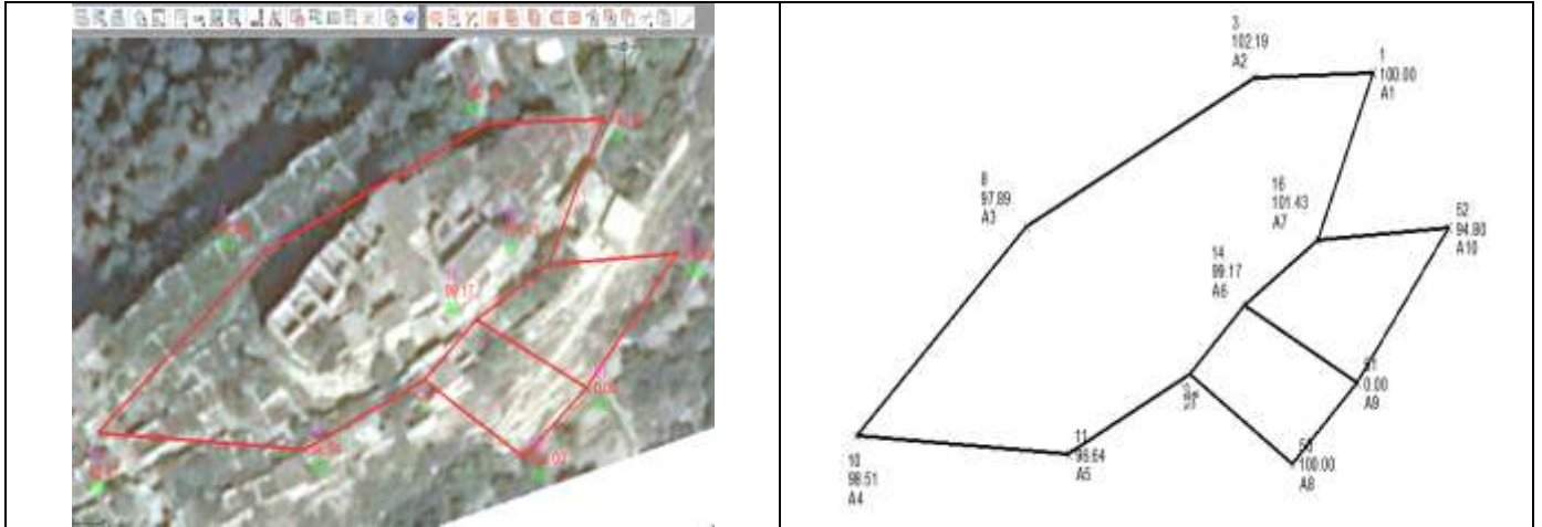
الشكل ( 2 ) شكل تخطيطي للشبكة الجيوديزية لقلعة الخوابي
