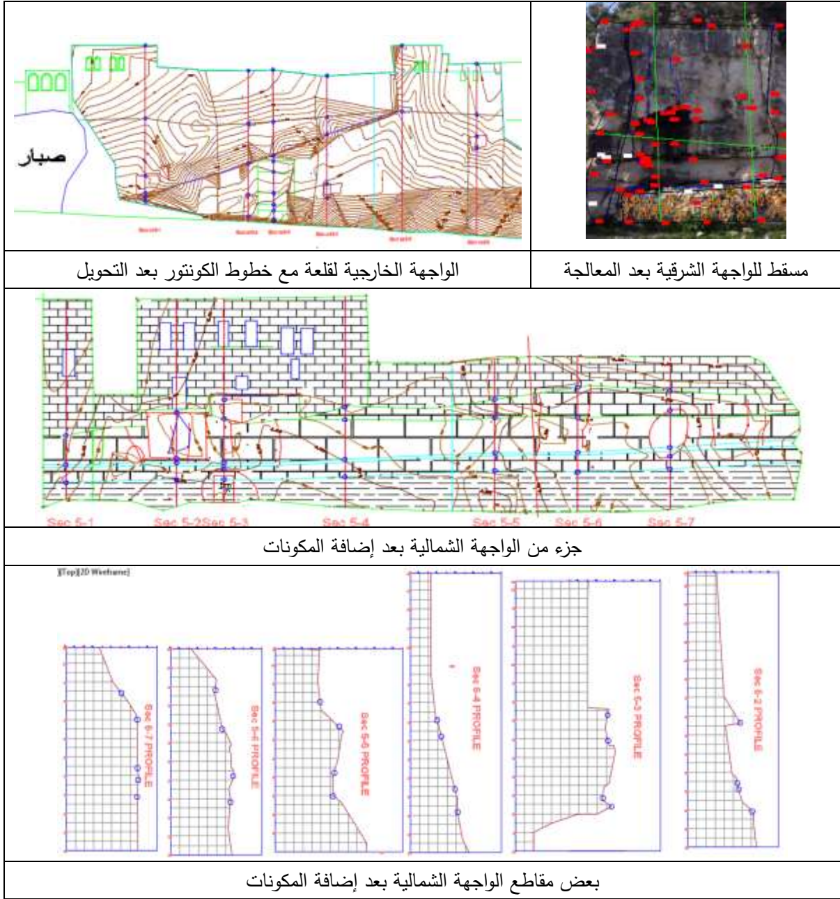
الشكل (10) المقاطع العرضية النهائية المنجزة
