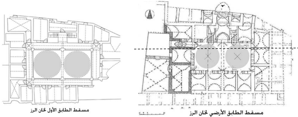
مخطط (7-8) مسقط الطابق الارضي والاول
