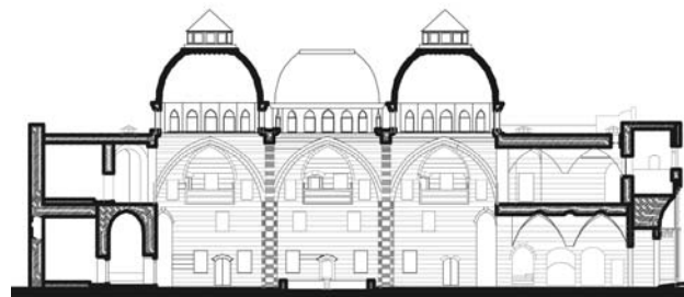
مخطط (6) مقطع في خان أسعد باشا مار من البوابة الرئيسية 3 [7]
