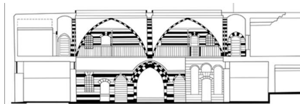
مخطط (9) مقطع في خان الرز مواز لشارع مدحت باشا
