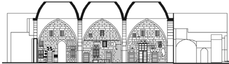
مخطط (25) مقطع في خان التتن عمودي على سوق الصاغة
