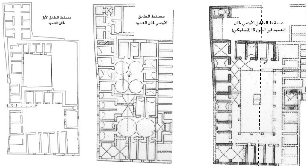
مخطط (13) خان العمود الطابق الأرضي القرن 16 مخطط (14-15) خان العمود اليوم الطابق الأرضي والطابق الأول
