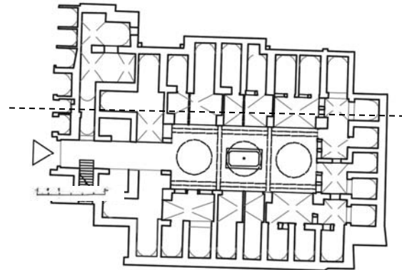
مسقط الطابق الأرضي لخان السفرجلاني
