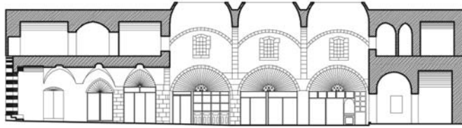
مخطط ( 22)مقطع في خان السفرجلاني عمودي على سوق الصاغة
