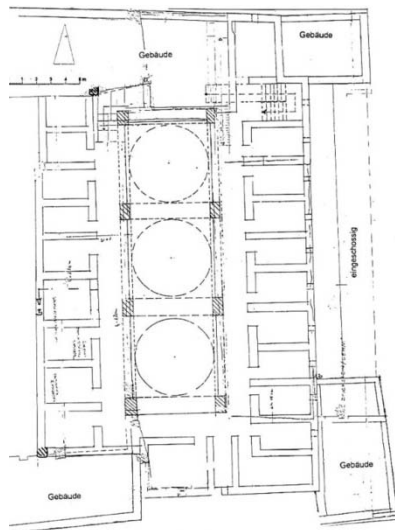
مسقط الطابق الأول خان السنوبر
