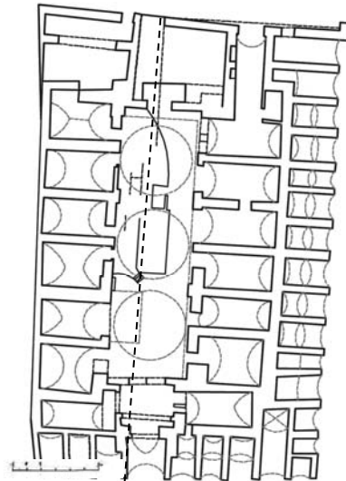
مسقط الطابق الأرضي خان السنوبر
