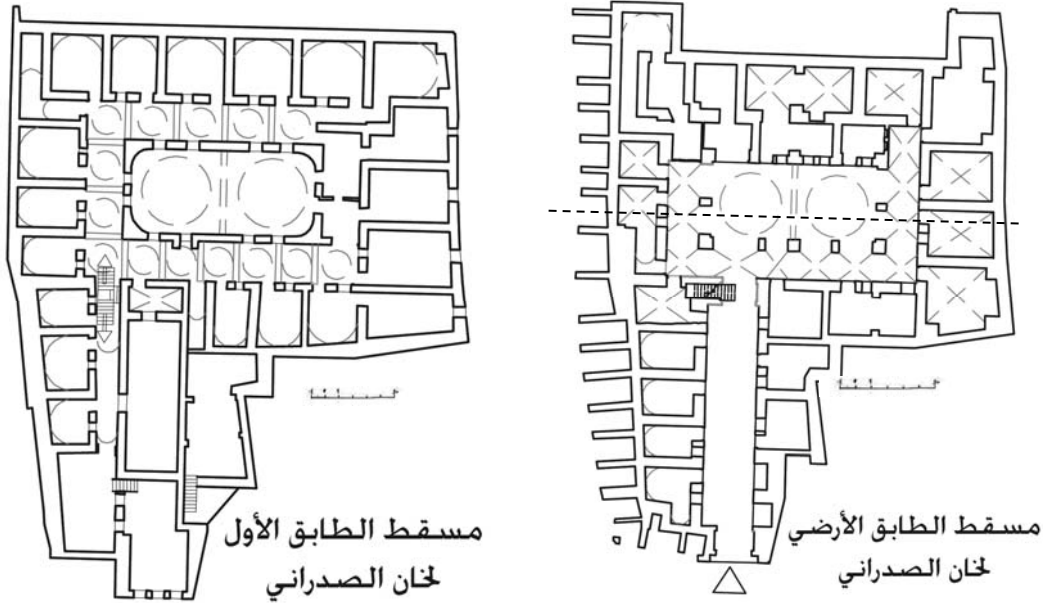
مخطط (17-18) مسقط الطابق الارضي والاول لخان الصدراني 11
