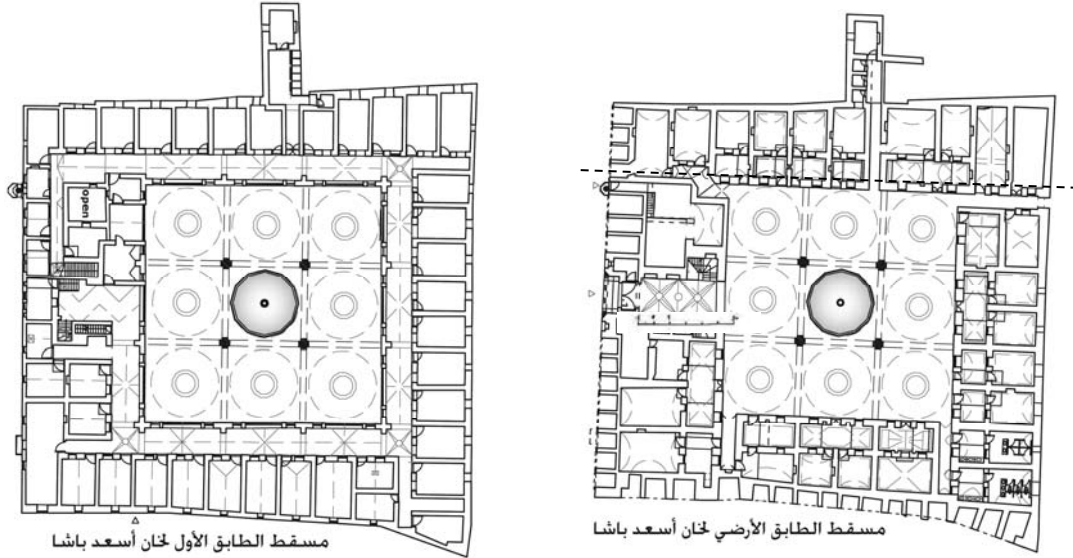
مخطط (4-5) مسقط الطابق الارضي والاول 3 [7]
