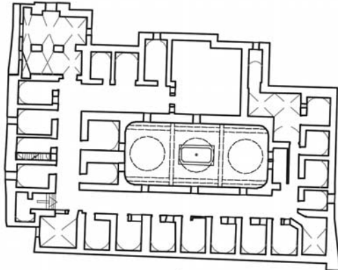
مسقط الطابق الأول لخان السفرجلاني
