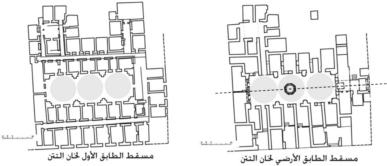
مخطط ( 23-24) مسقط خان التتن الطابق الارضي والأول
